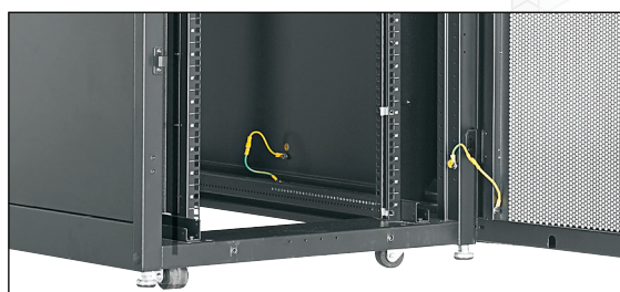
Linki uziemiające na drzwiach i panelach bocznych połączone z konstrukcją szafy dla ochrony sprzętu oraz personelu
