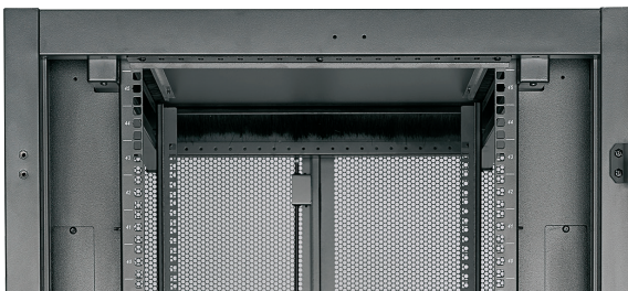
Zintegrowane pionowe panele zaślepiające w szafie o szerokości 800mm oferują 4 pionowe otwory 1U, które poprawiają wykorzystanie powierzchni szafy nawet o 10%
